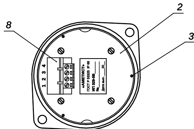
Блок извещателя. Вид со стороны контактов
