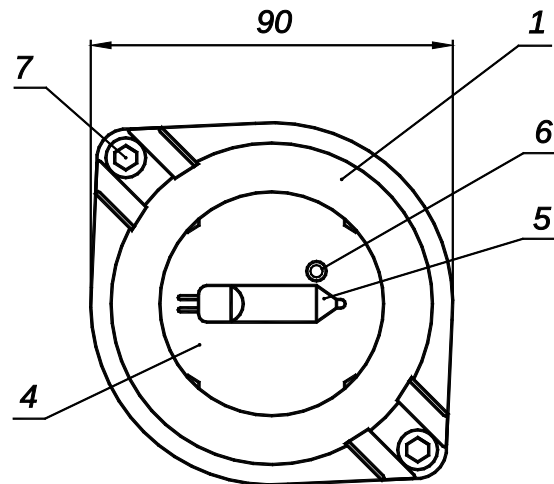
Блок извещателя. Вид со стороны контактов
