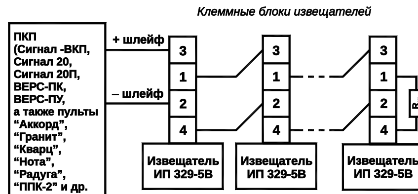
Пример схемы подключения извещателей ИП 329-5В к двухпроводной системе пожарной сигнализации
